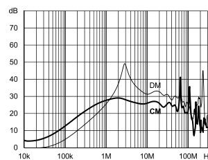
10Aタイプ
