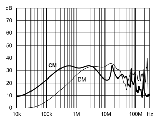
4Aタイプ
